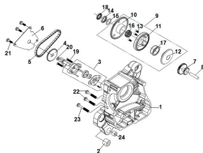
E07 AC GEN. ASSY
