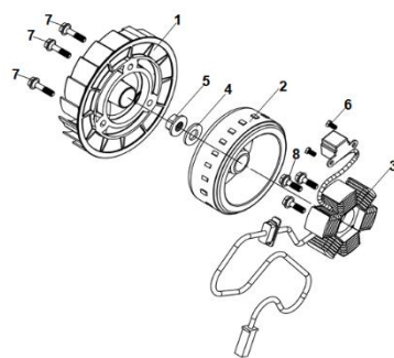
E07 AC GEN. ASSY
